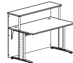
BALÇÃO 800 X 800 X 1100 | 1600 X 800 X 1100 1200 X 800 X 1100 | 1800 X 800 X 1100 1400 X 800 X 1100
