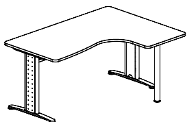
COMPACTO "A" 1400 X 1200 X 740 ESQ. | 1400 X 1200 X 740 DIR. 1600 X 1200 X 740 ESQ. | 1600 X 1200 X 740 DIR. 1800 X 1200 X 740 ESQ. | 1800 X 1200 X 740 DIR.
